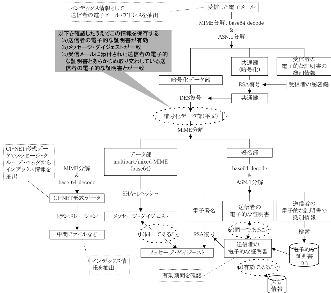
図B.VIII-13 保管処理の概要イメージ
