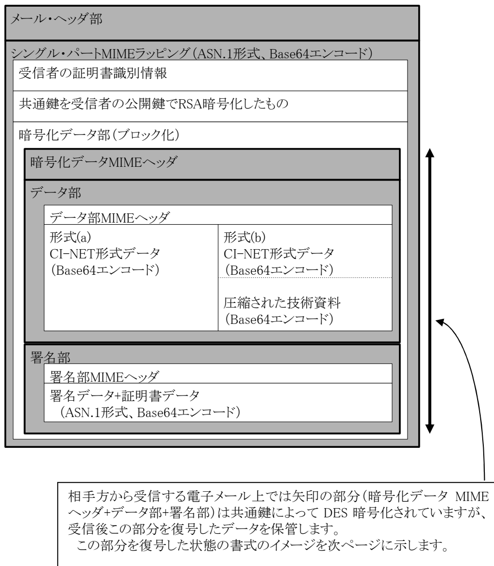
図B.VIII-11 CI-NET LiteS の電子メールの書式と保管する電磁的記録の範囲
