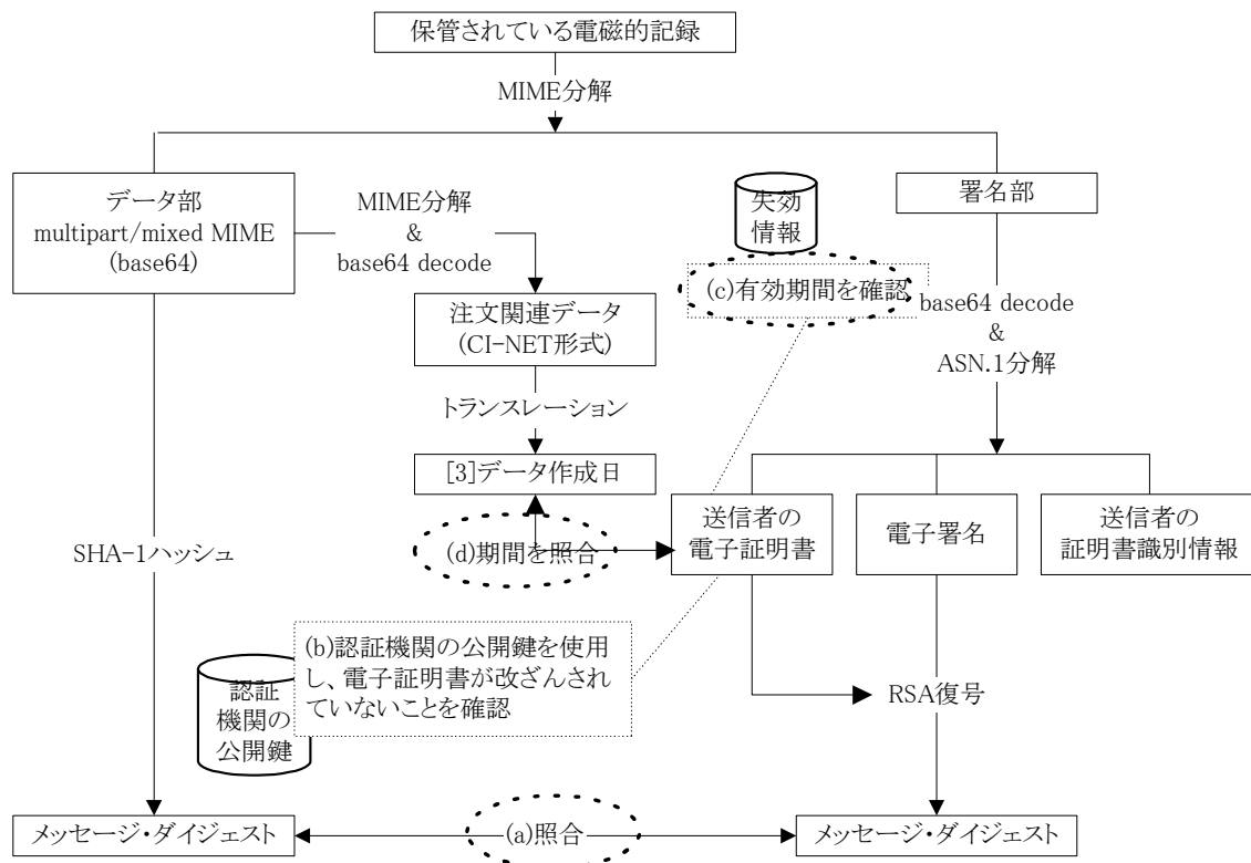
図B.VIII-15 改ざんされていないことの確認処理の概要イメージ
