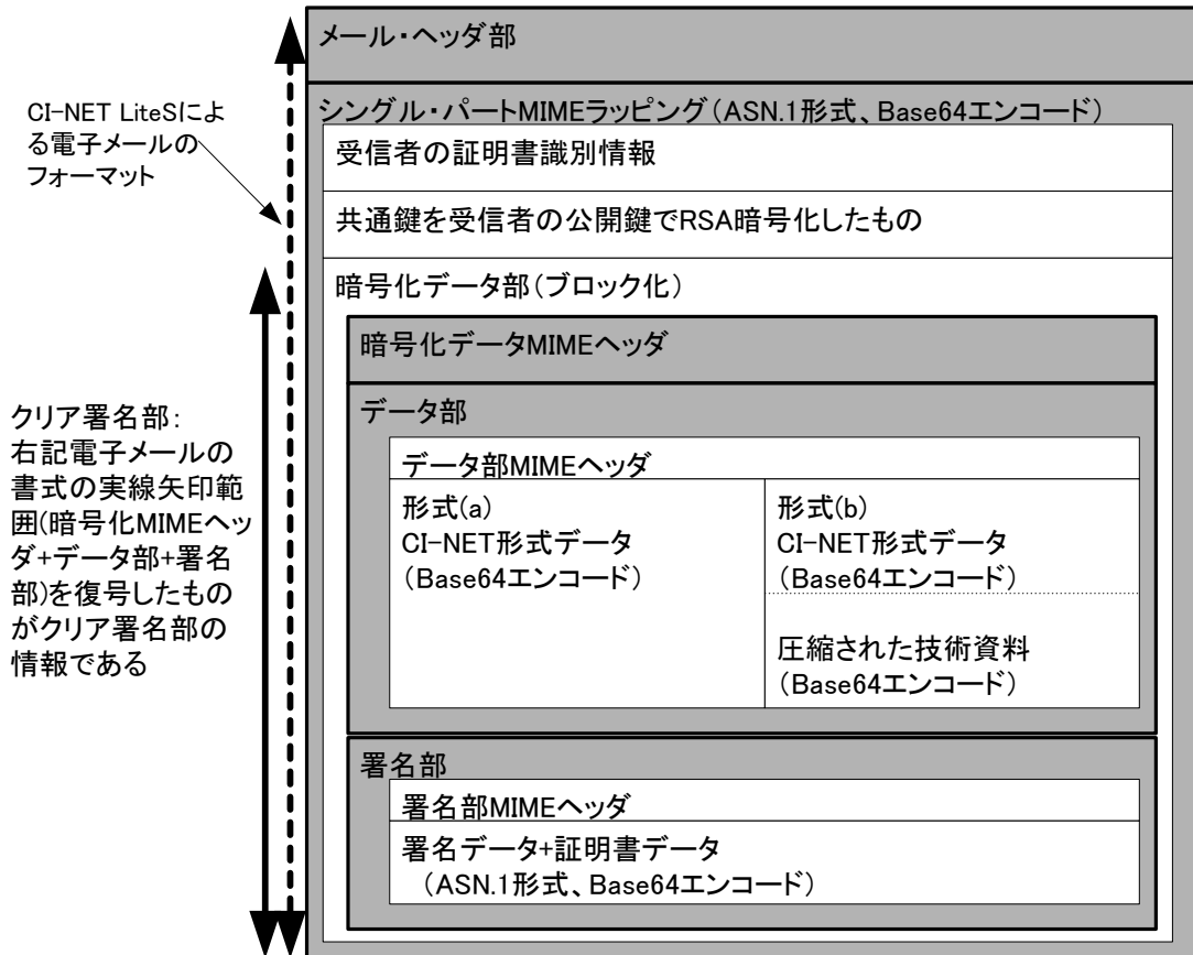
図B.VIII-20 クリア署名部
