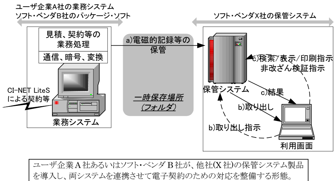
図B.VIII-17 本資料が前提とするシステムの形態
