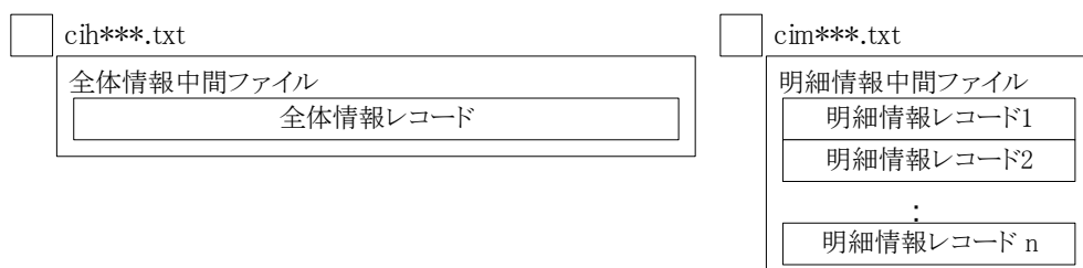
図 B. II - 8 CI-NET LiteS 互換中間ファイルの全体情報中間ファイルと明細情報中間ファイルの関係
