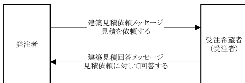
図 B. II - 1 建築見積業務 EDI のデータ交換手順
