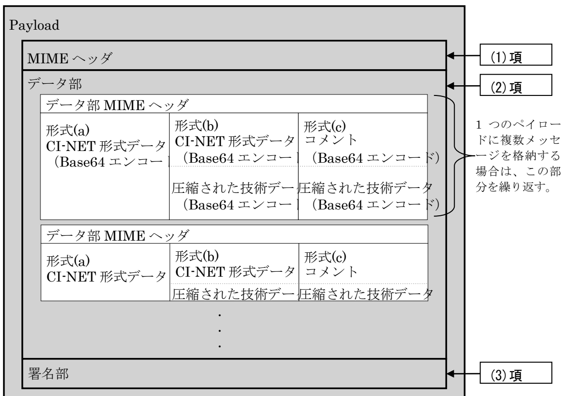
図 A- 18 ペイロードコンテナへのデータ格納構造の概要
