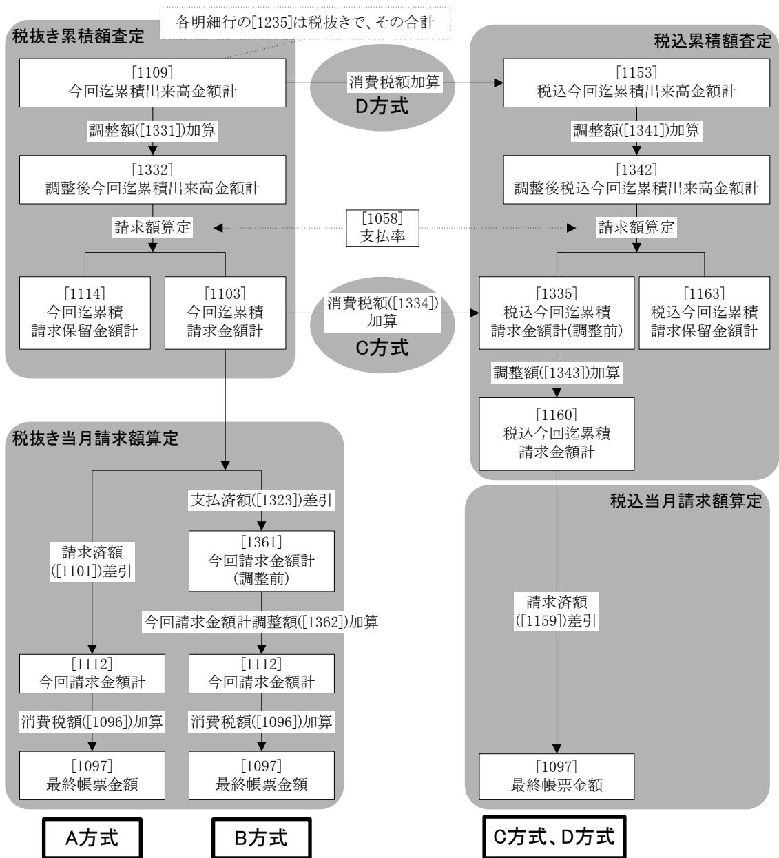
図 B.VII- 12 全体情報部分(鑑)の出来高金額、請求金額算定方法
