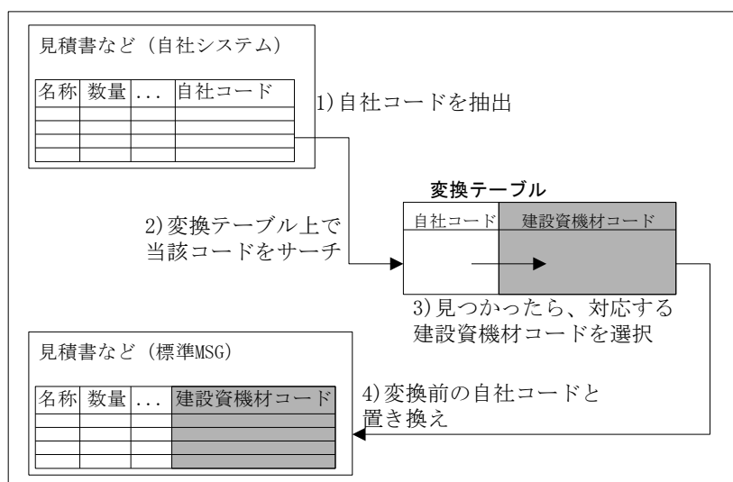
図 B.Ⅲ- 8 コード送信側変換結果コードの設定方法
