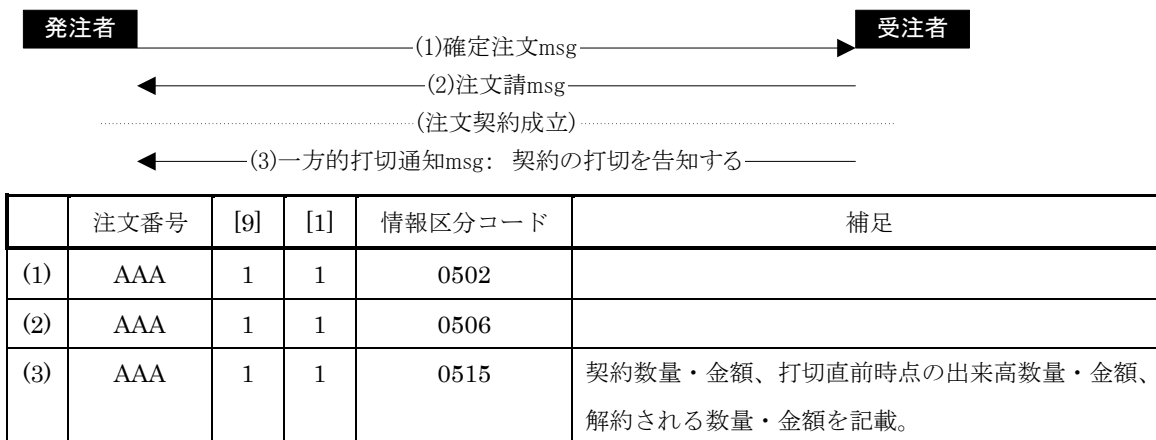
図 B.VI- 10 受注者からの一方的打切通知の処理フロー
