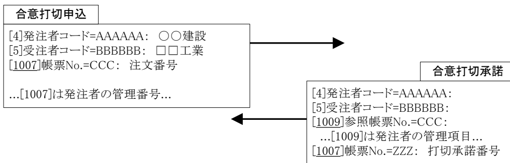
図 B.VII- 13 [1007]帳票 No.と[1009]参照帳票 No.による合意打切申込と承諾の対応づけ
