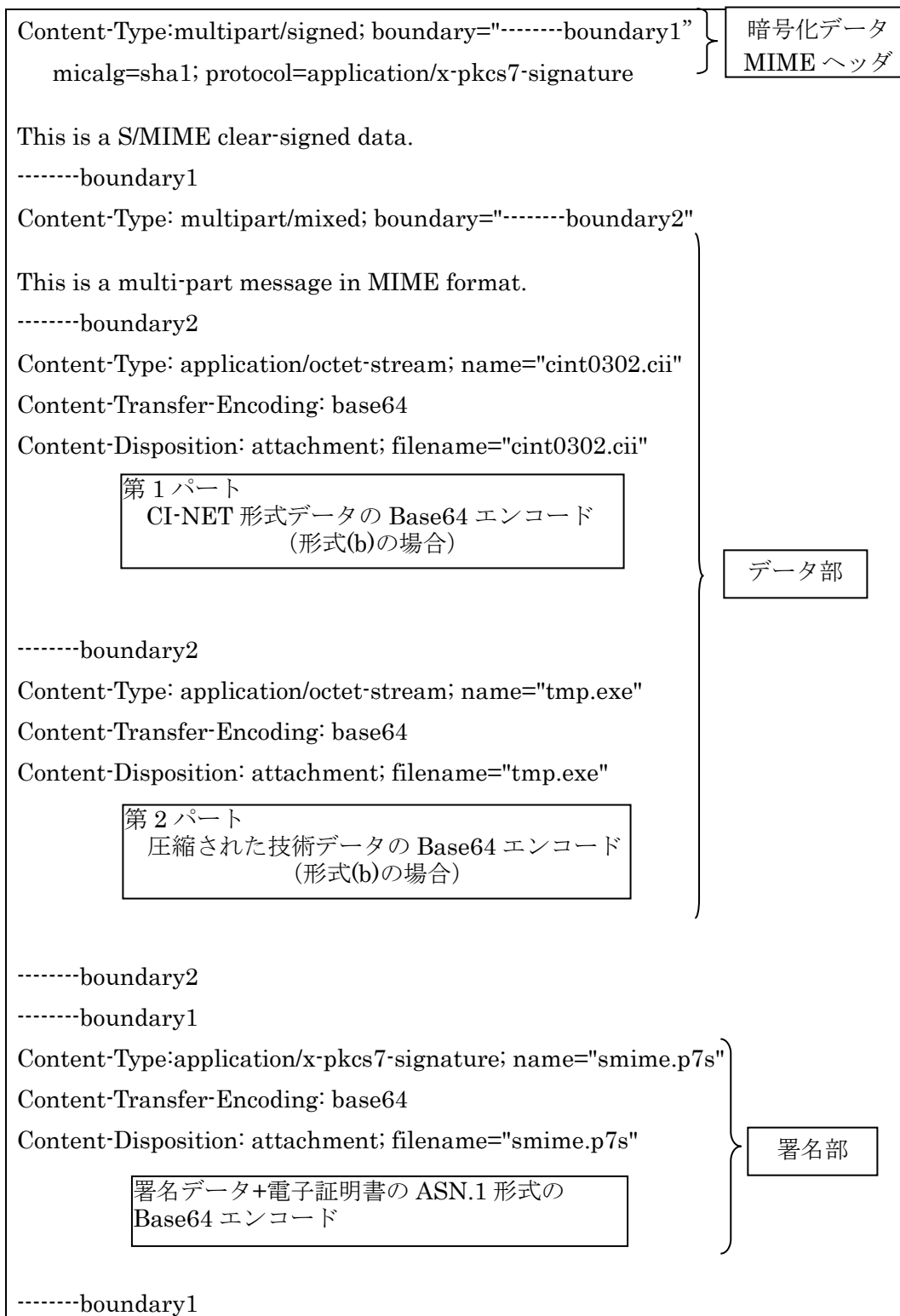
図 A- 12 暗号化データ部の記述例（平文状態のもの）
