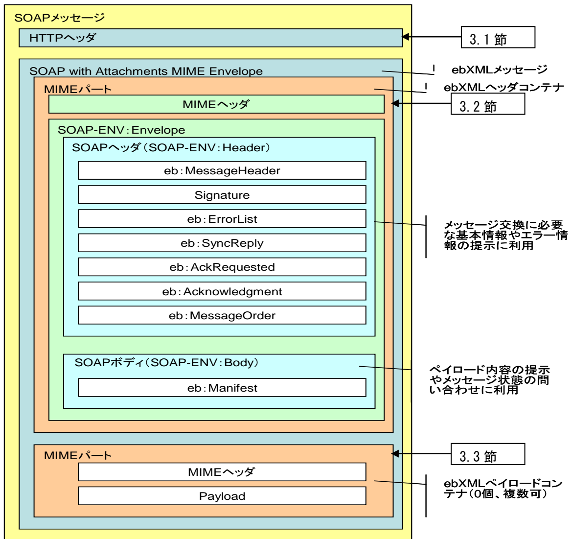
図 A-17 ebMS メッセージへのデータ格納構造の概要
