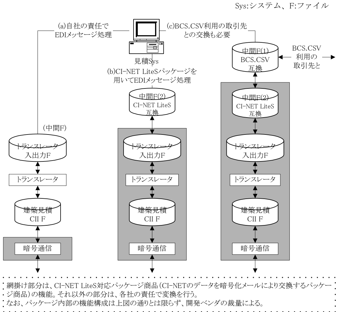
図 B. II - 6 建築見積業務の中間ファイルの種類
