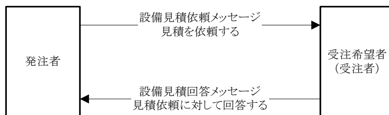
図 B.Ⅲ-1 設備見積業務 EDI のデータ交換手順
