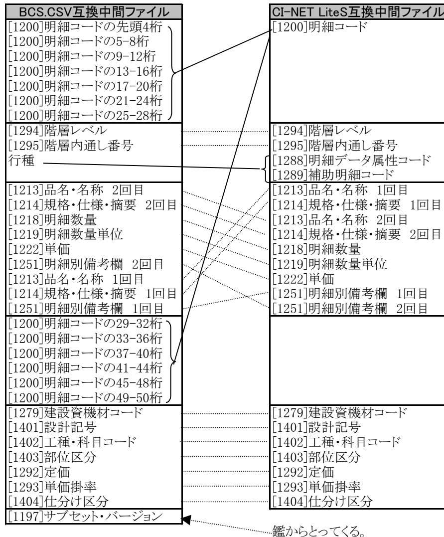
図 B. II - 10 明細情報中間ファイルの相互変換
