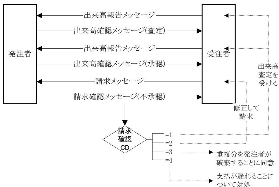
図 B.VII- 1 請求不承認の場合の手続き
