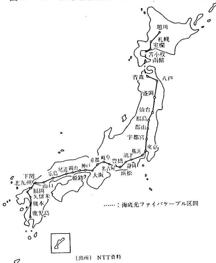
図 2 - 2 日本縦貫光ファイバーケーブル伝送路
