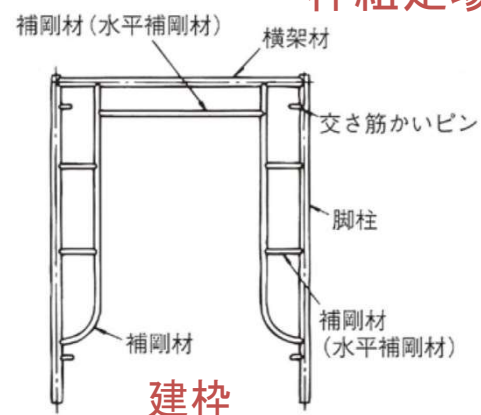
枠組足場(ビティ)
