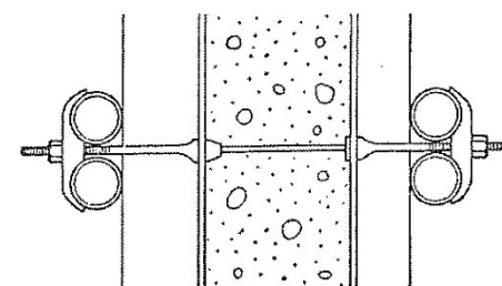
片面打ち放し 片面モルタル仕上げBC型
