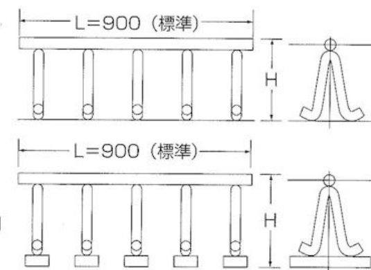
鋼製連続サポート 床スラブ下端筋用
