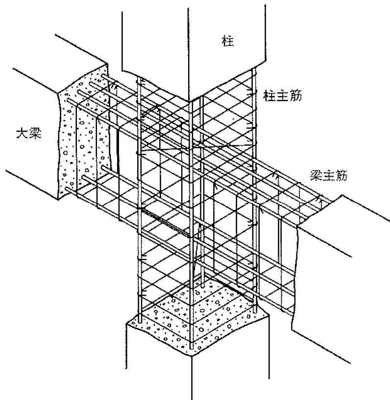
通常の内柱・梁接合部
