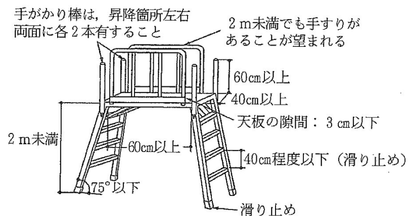
移動式室内足場
