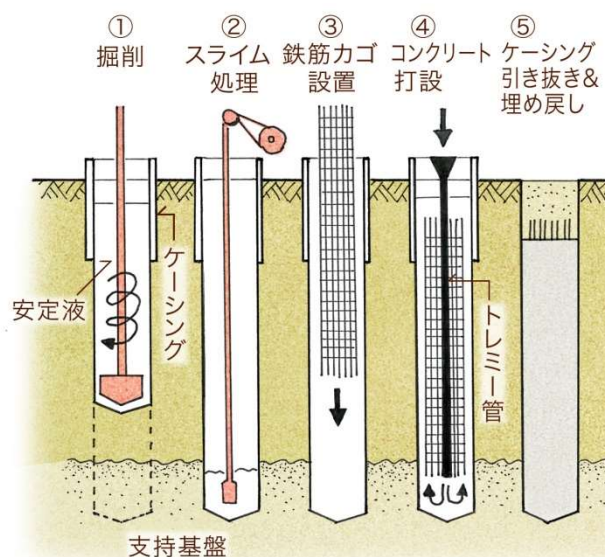
《場所打ち杭 施工手順》
