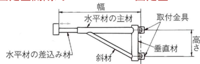
固定型開閉式
