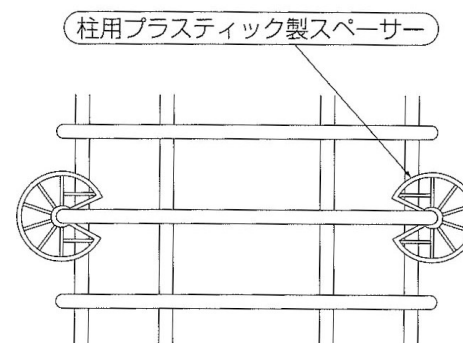
壁・柱・梁側用プラスチック製スペーサー
