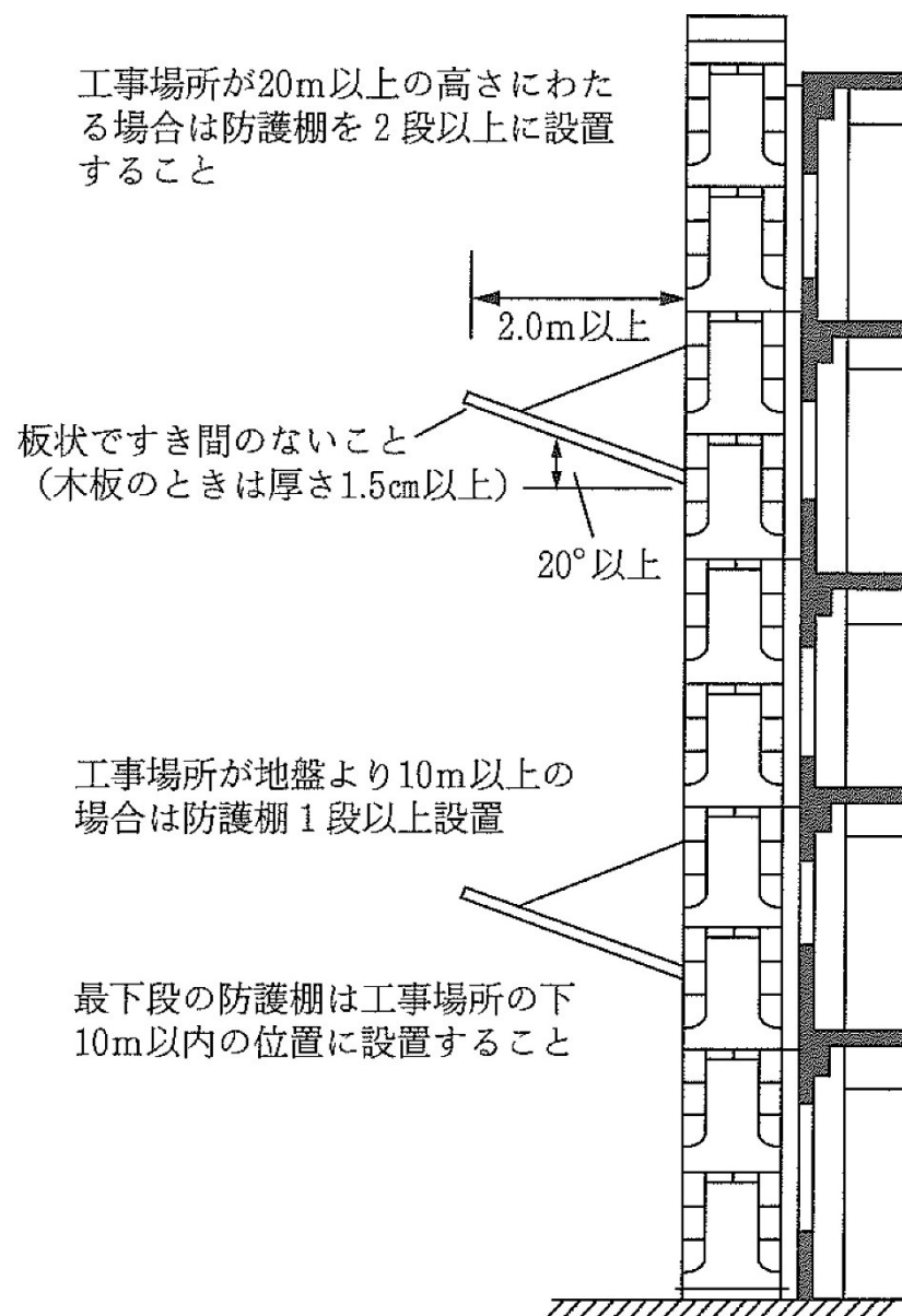
防護棚(朝顔)の取付け例
