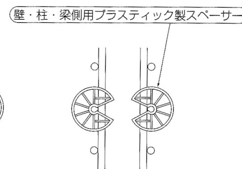
柱用プラスチック製スペーサー
