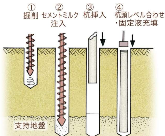
《既製杭 施工手順》
