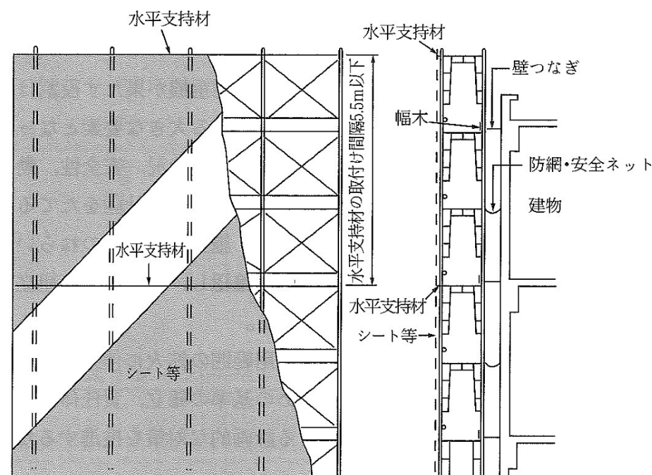
工事用シートの取付け例
