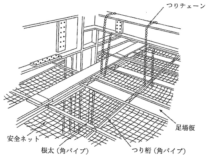
つり柵足場
