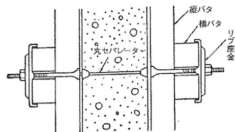
打ち放し用B型
