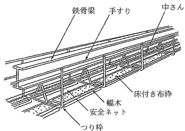
つり桟足場
