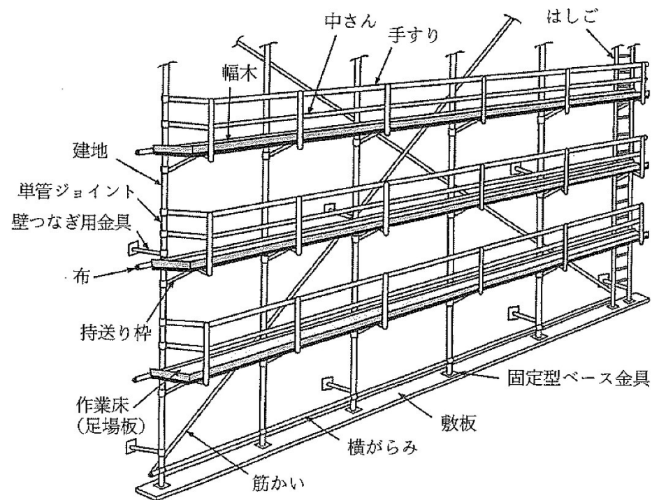
ブラケット側足場
