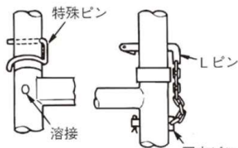
ピン差し式
