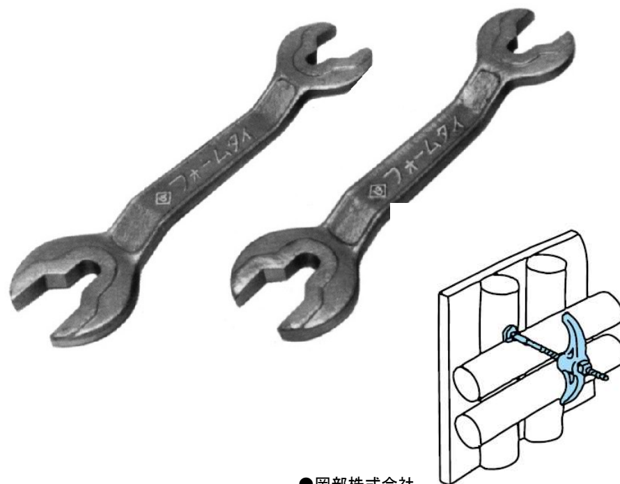
フォームタイ回し(フォームタイスパナ)
