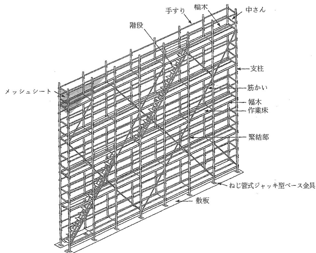
くさび緊結式足場(ビケ)
