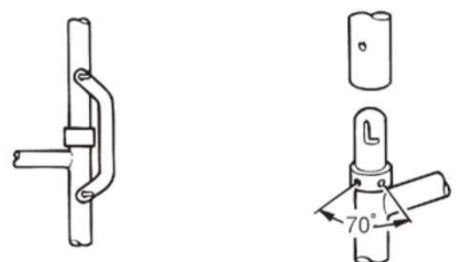
アームロック式
