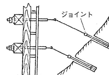
ロックボルト締付図
