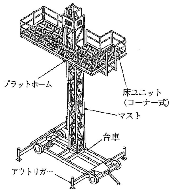
移動式昇降足場
