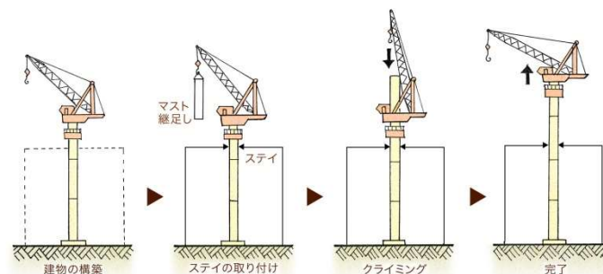
■ マストクライミング方式
