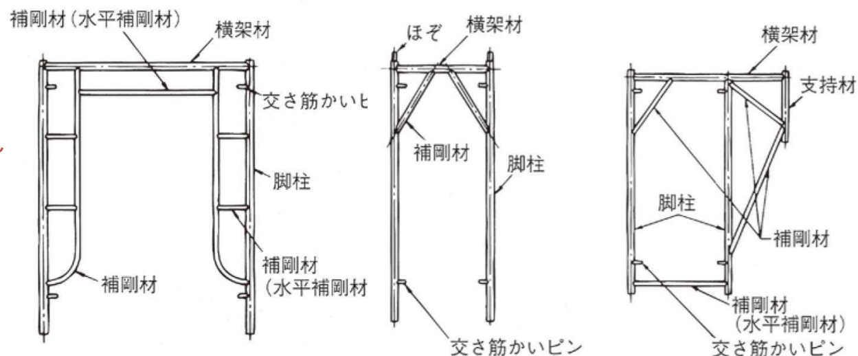
標準枠
