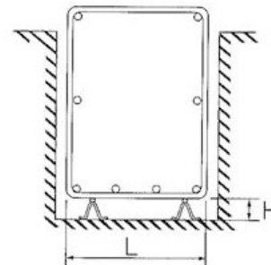
鋼製連続サポート 床スラブ下端筋用
