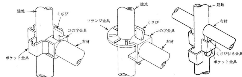
緊結方式
