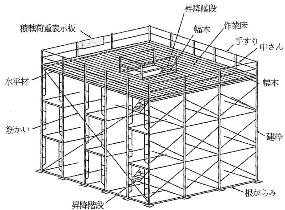
棚足場
