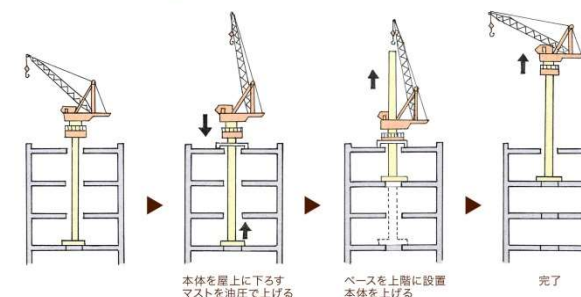
■ フロアクライミング方式
