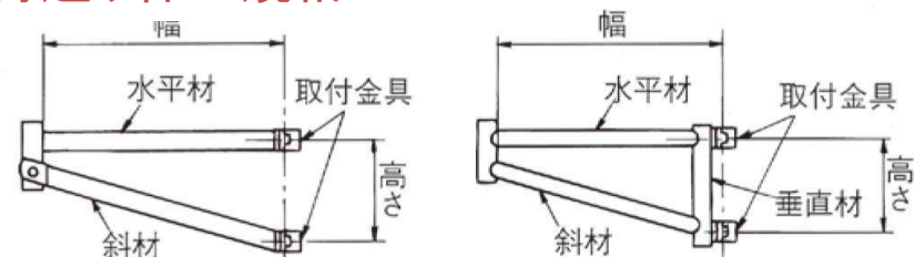
固定型開閉式
