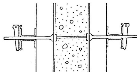
モルタル仕上げC型
