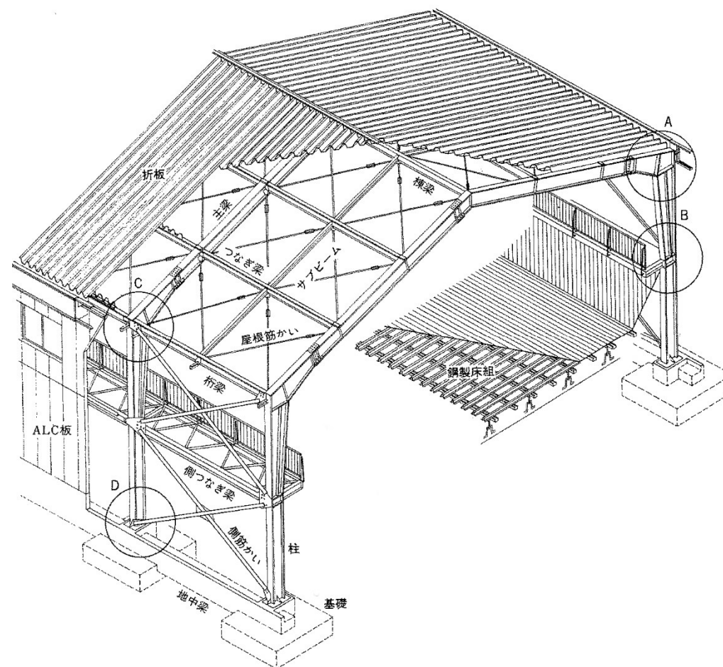
【長方形ラーメン構造】
