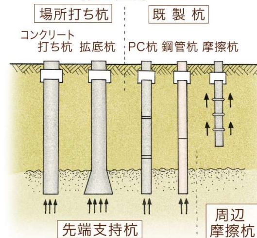
《杭の種類》
